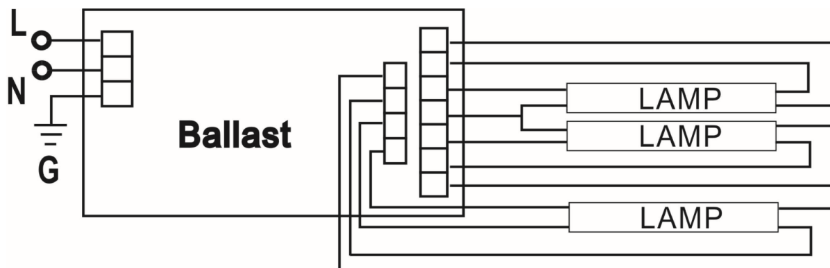
結線図
